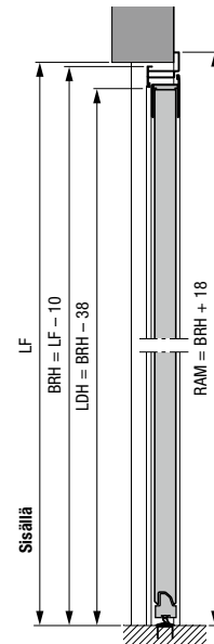
Sivuovi alumiinisella kulmakarmilla, profiilityyppi 2 Ulkopuolella oleva rajoitin
