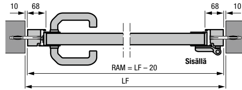
Alumiinisella karmilla varustettu sivuovi, profiilityyppi 2 Asennus aukkoon
