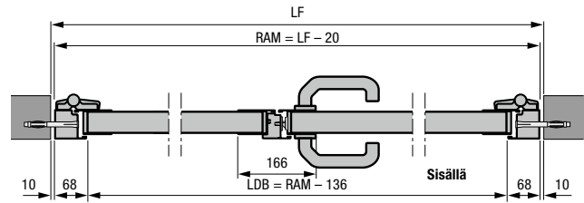
2-lehtinen sivuovi ja alumiininen suorakaidekarmi, profiilityyppi 2 Asennus aukkoon
